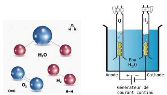
Les molécules de dihydrogène, d'oxygène et d'eau et l'électrolyse de l'eau
